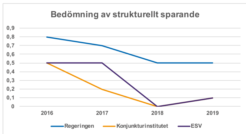
Figur 5. Jämförelse av hur regeringen, KI och ESV bedömer storleken på det strukturella sparandet. Siffrorna anger procent av BNP.
