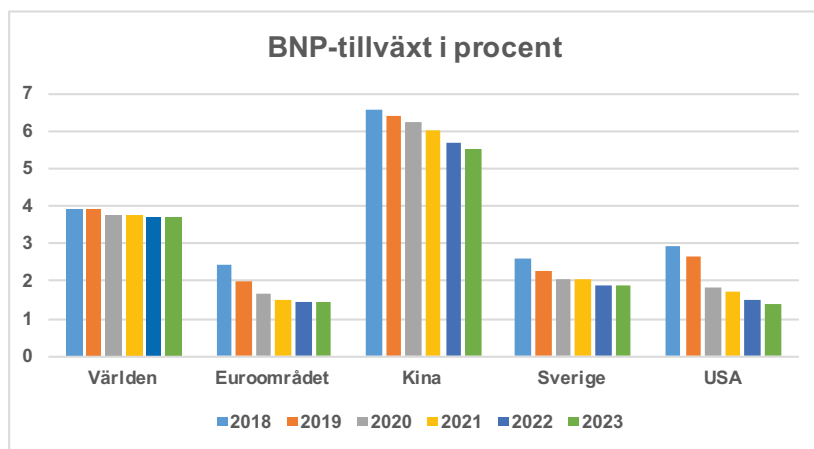
Figur 1. Tillväxtutveckling (2018–2023) i världen, euroområdet, Kina, Sverige och USA (källa: IMF).
